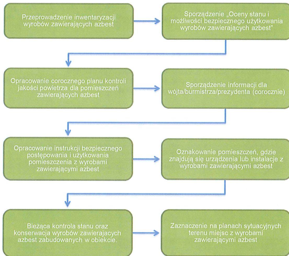
Rysunek 3. Schemat procedury dotyczącej obowiązków i postępowania właścicieli i zarządców przy użytkowaniu obiektów i terenów z wyrobami zawierającymi azbest
